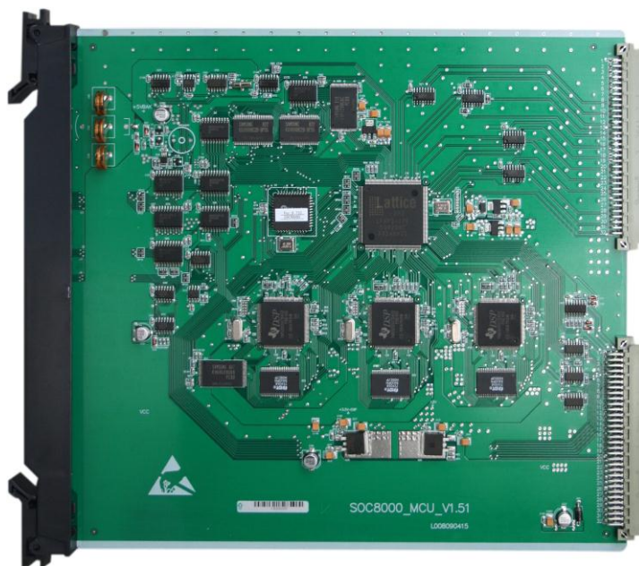
图 3-5 MCU 主控板
