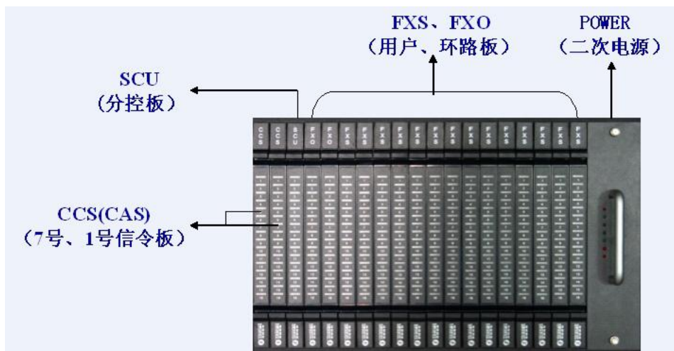
图 3-4 副框示意图
